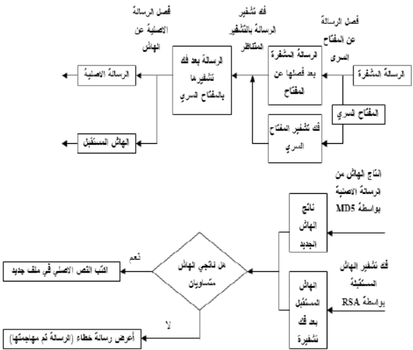
شكل (٢) تسلسل عملية فك التشفير بواسطة خوارزمية PGP
